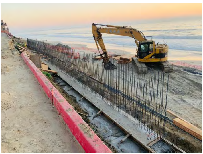
0+000 a 0+300 Terracerías, pilotes y muro de contención
